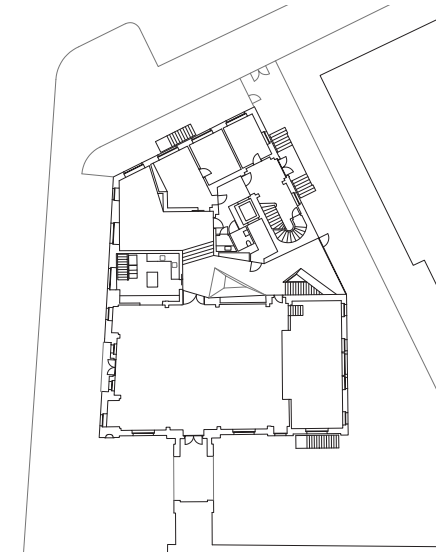
Erdgeschoss
