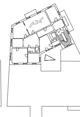
1. Obergeschoss
